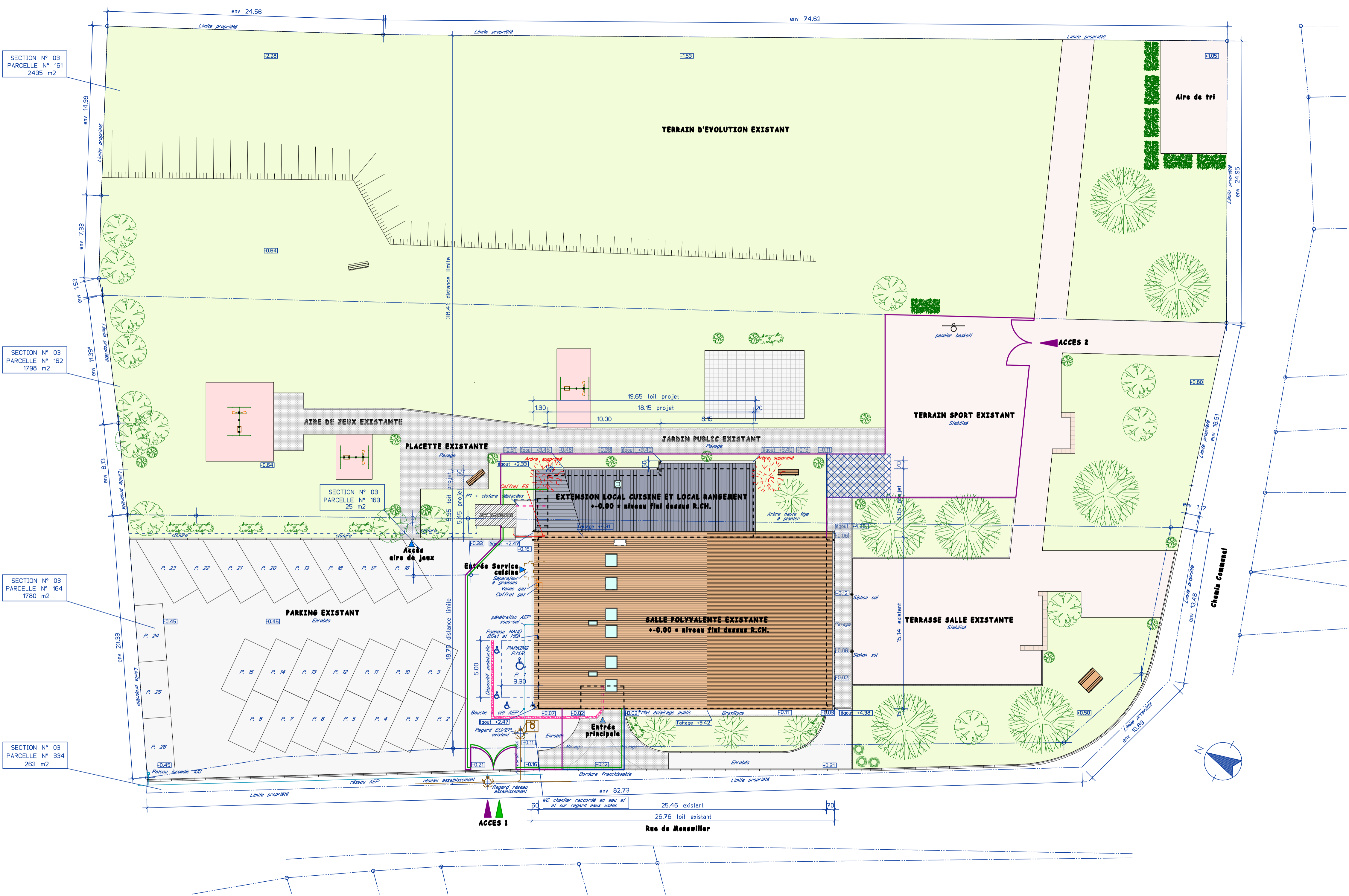
PLAN MASSE 1/200°
